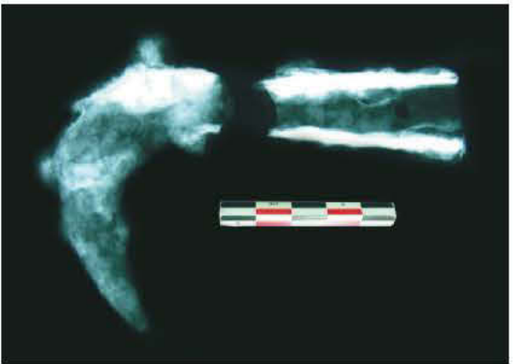
Radiographie d'une serpe gauloise retrouvée sur le site de la Tourelle (© Arc'Antique).
